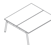
BOM35 1800 / 1610 / 740 74 kg
